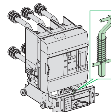
Механизм блокировки двери отсека выключателя
