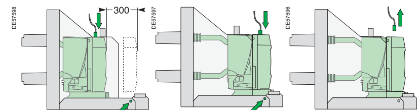
Положение «Рабочее» Положение «Испытание» Положение «Выкочен»
